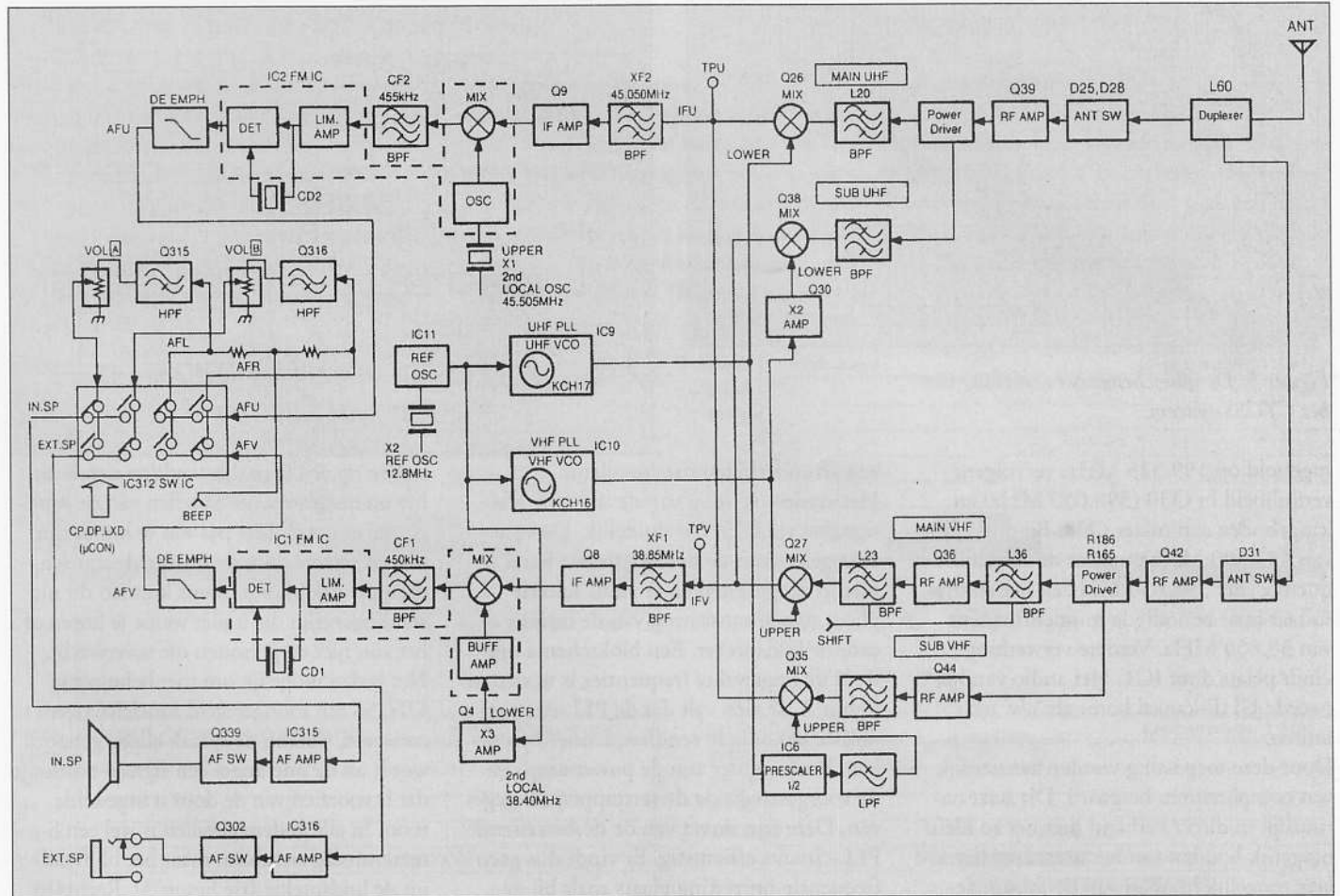
Figuur 1: De blokschematische opbouw van het ontvangste gedeelte.
